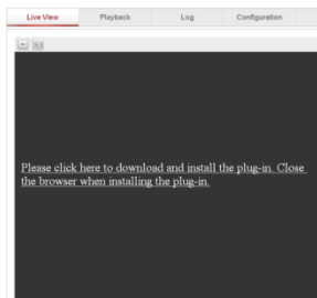
Figure 4-2 Stáhnutí pluginu
