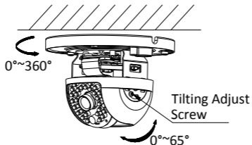
Figure 2-5 Typ kamery I Nastavení úhlu
