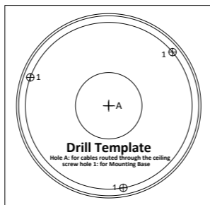
Figure 2-1 Vrtací šablona
