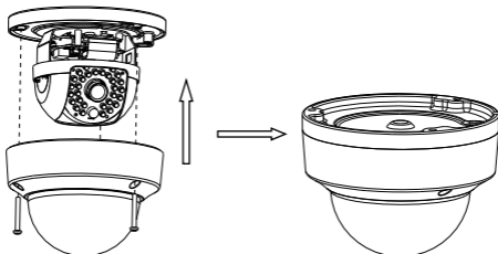
Figure 2-7 Namontování kopule
