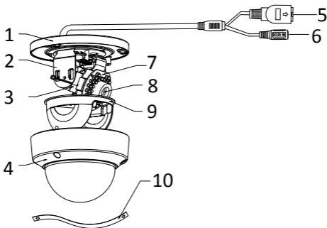
Figure 1-1 Přehled typů I kamer
