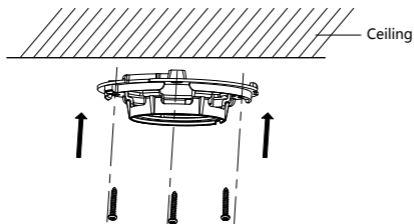
Obrázek 2-4 Zajištění montáže na stropě
