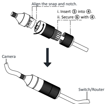
Obrázek 2-23 Instalace vodovzdorného příslušenství
