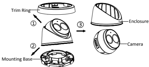
Obrázek 2-15 Demontáž kamery
