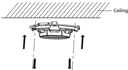
Obrázek 2-12 Připevnění kamery ke stropu
