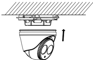
Obrázek 2-5 Připevnění kamery k montážní podložce
