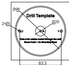
Obrázek 2-10 Vrtací šablona
