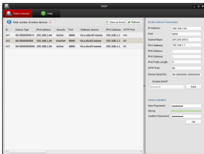
Obrázek 3-4 Rozhraní SADP
