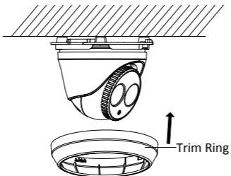
Obrázek 2-8 Instalace zkoseného prstence
