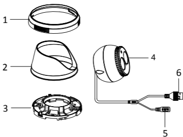
Obrázek 1-2 Přehled o kameře věžičkového typu II
