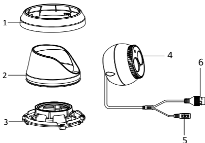
Obrázek 1-1 Přehled o kameře věžičkového typu I
