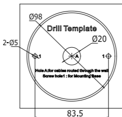
Obrázek 2-18 Vrtací šablona
