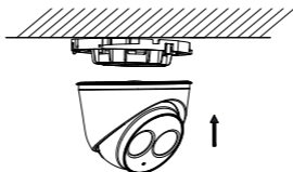
Obrázek 2-20 Instalace kamery
