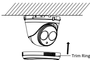
Obrázek 2-14 Instalace zkoseného prstence
