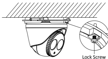
Obrázek 2-6 Uvolnění pojistného šroubu
