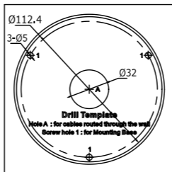
Obrázek 2-2 Vrtací šablona
