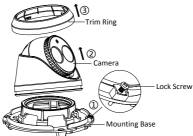
Obrázek 2-1 Demontáž kamery
