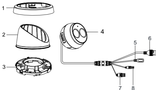
Obrázek 1-3 Přehled o kameře věžičkového typu III
