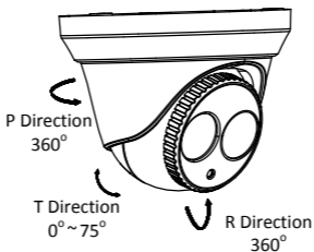
Obrázek 2-7 Nastavení objektivu
