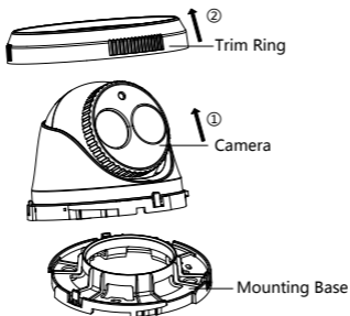
Obrázek 2-9 Demontáž kamery
