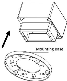
Obrázek 2-8 Stropní montáž
