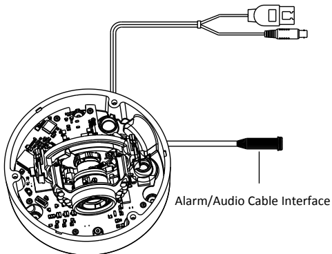
Obrázek 1-2 Rozhraní audio/výstražného signálu
