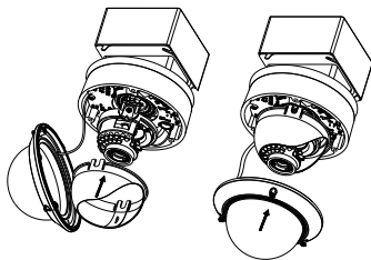
Obrázek 2-10 Kopuli zajistěte
