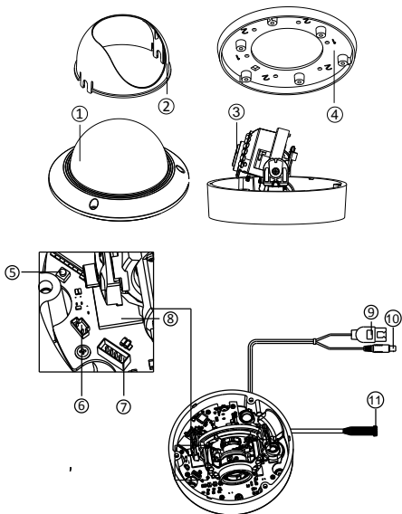
Obrázek 1-1 Přehled
