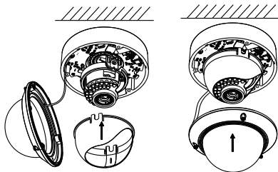
Obrázek 2-4 Zajistěte černou vložku a kopuli
