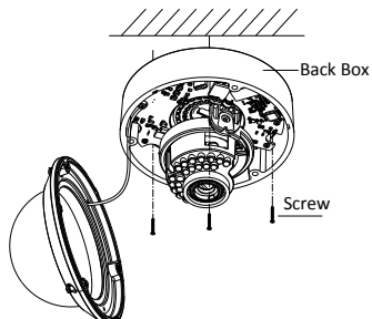
Obrázek 2-3 Kameru zajistěte
