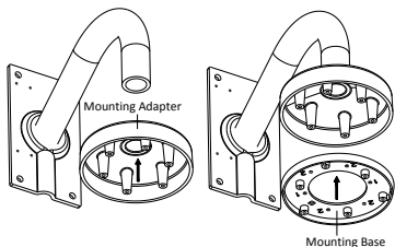
Obrázek 2-11 Instalace montážní podložky
