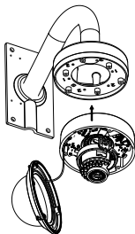
Obrázek 2-12 Kameru zajistěte
