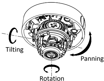
Obrázek 2-14 3osá aretace
