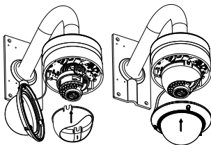
Obrázek 2-13 Zajistěte černou vložku a kopuli
