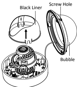
Obrázek 2-1 Odstraňte kopuli a černou vložku.
