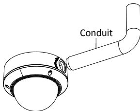
Obrázek 2-6 Nainstalujte kabelovod do kameru
