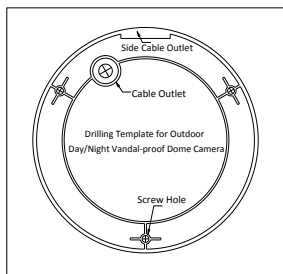
Obrázek 2-2 Vrtací šablona
