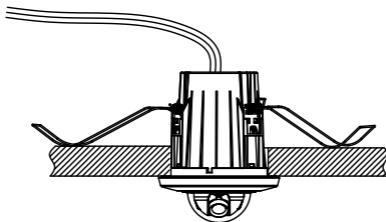
Obrázek 2-6 Dokončení instalace
