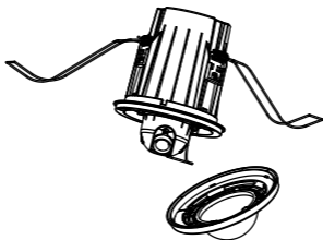
Obrázek 2-2 Demontáž kopule
