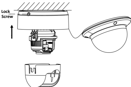
Obrázek 2-4 Instalace montážní podložky
