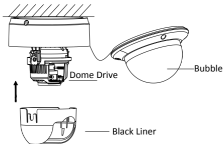
Obrázek 2-8 Instalace černé vložky a kopule
