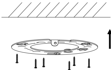
Obrázek 2-3 Nainstalujte podložku adaptéru
