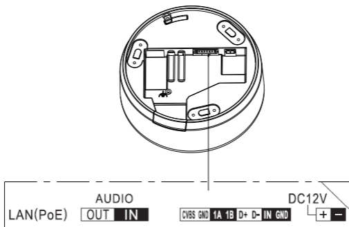
Obrázek 1-4 Přehled (4)
