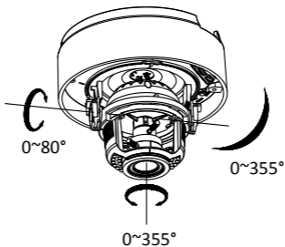
Obrázek 2-5 3osá aretace
