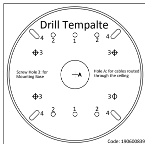
Obrázek 2-1 Vrtací šablona
