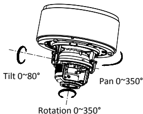
Obrázek 2-4 3osá aretace
