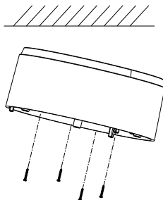
Obrázek 2-9 Instalace montážní podložky
