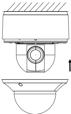
Obrázek 2-10 Instalace pohonu kopule
