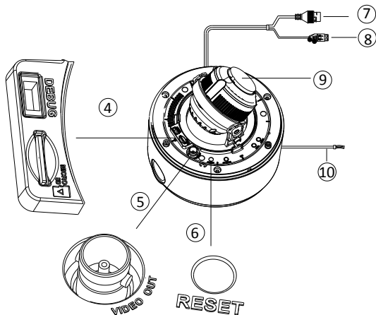
Obrázek 1-2 Přehled (2) o kameře kupulového typu II
