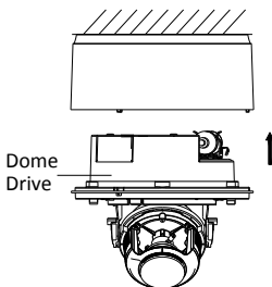
Obrázek 2-3 Instalace pohonu kopule
