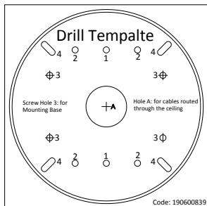
Obrázek 2-8 Vrtací šablona
