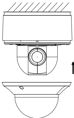
Obrázek 2-12 Instalace kopule
