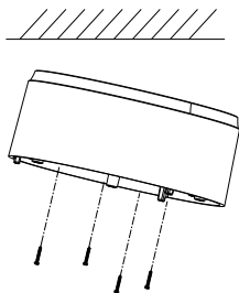
Obrázek 2-2 Instalace montážní podložky
