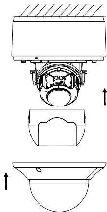
Obrázek 2-6 Instalace černé vložky a kopule
