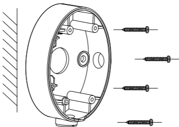
Obrázek 2-6 Instalace rozvodné krabice
