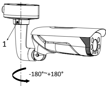
Obrázek 2-9 Nastavení úhlu panorámování
