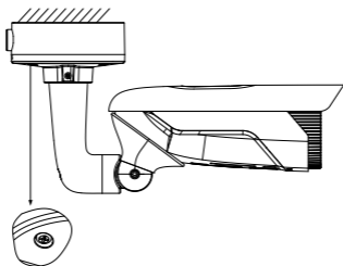
Obrázek 2-4 Dotáhněte pojistný šroub
