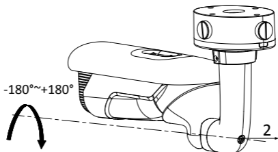
Obrázek 2-10 Nastavení úhlu naklápění
