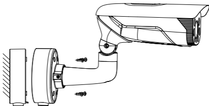
Obrázek 2-7 Instalace kamery
