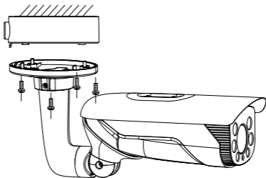
Obrázek 2-3 Instalace kamery
