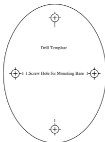
Obrázek 2-1 Vrtací šablona
